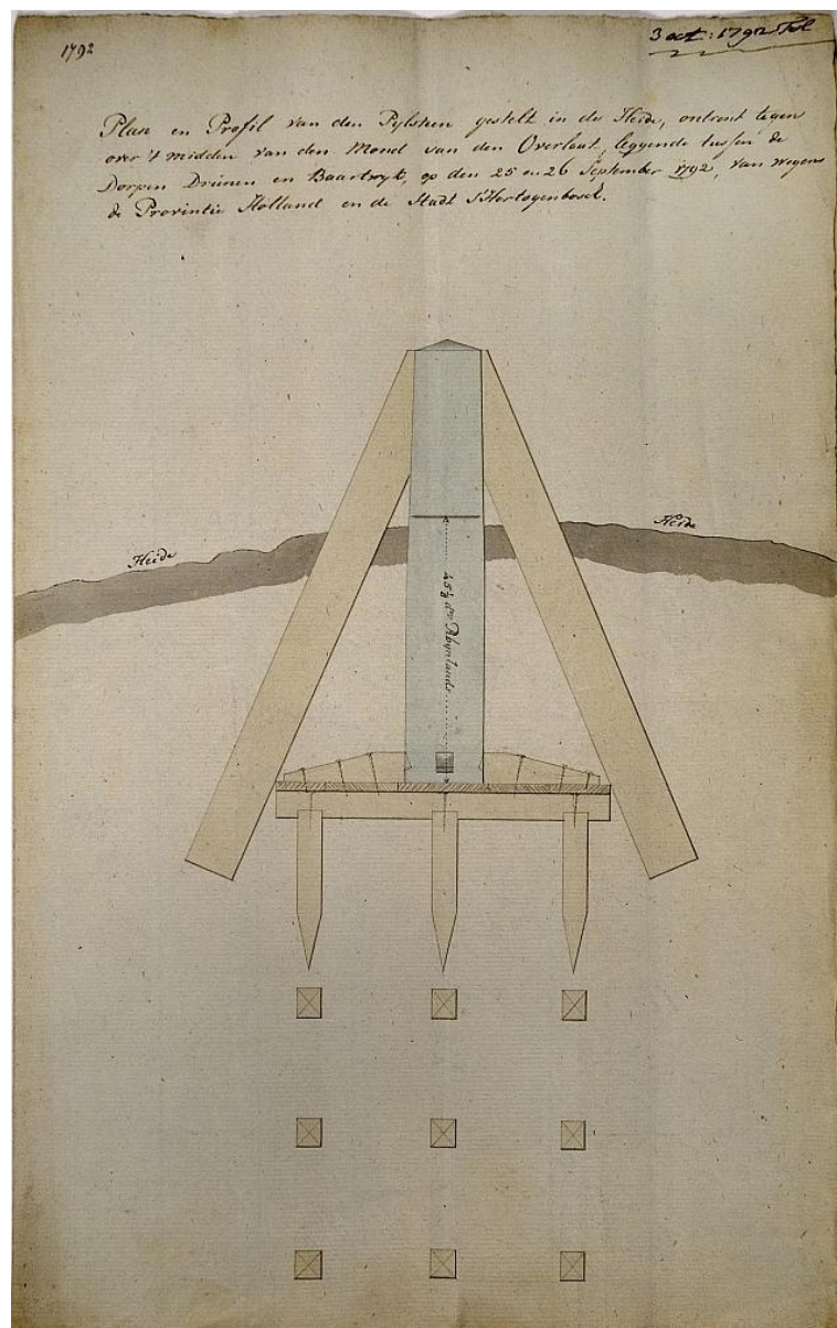
Pijlsteen bestemd voor de heide tussen Drunen en Baardwijk (Baardwijkse Overlaat). Tekening van Hendrik Verhees. (Bron: 10)
