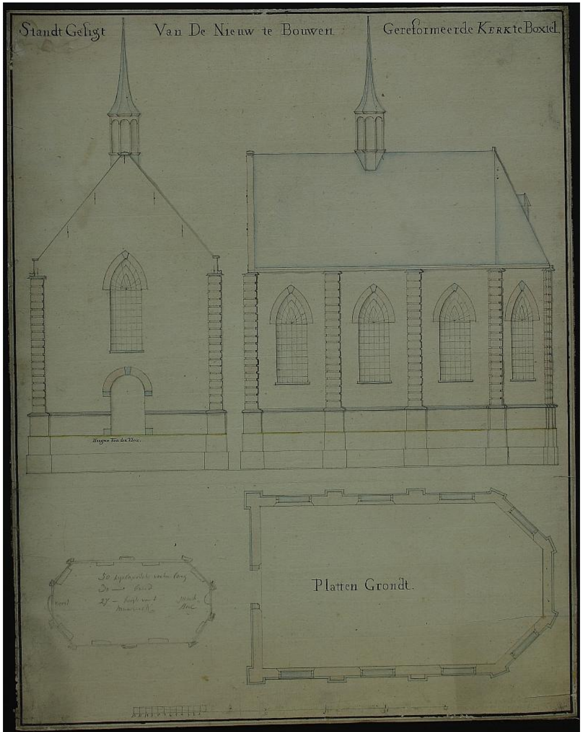
Tekening inzake ontwerp voor een nieuwe kerk voor de Protestantse Gemeente te Boxtel. Hendrik Verhees, 1812. De linksonder in geschetste omtrek van een kleinere, daadwerkelijk gerealiseerde, variant op het oorspronkelijke plan, mogelijk van de hand van Hendrik Verhees. (Bron: 5)
