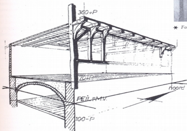
* Reconstructieschets van houtconstructie en keldergewelf.
