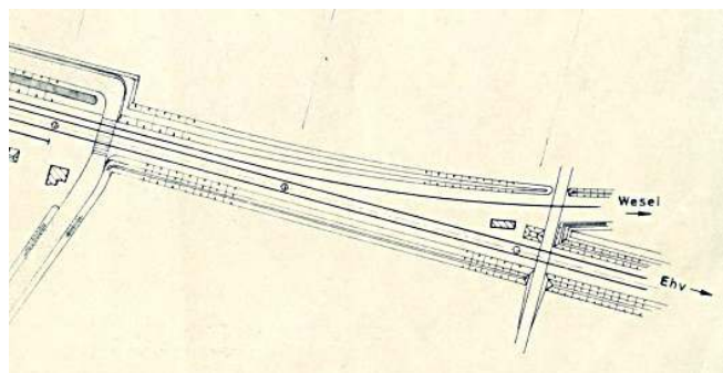
Aansluiting spoor uit Wesel op Boxtels emplacement
