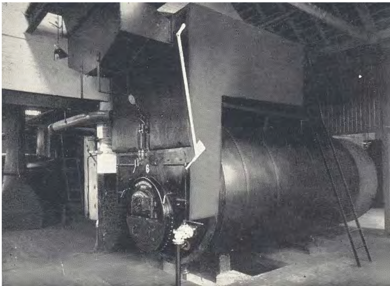
De in 1931 bijgeplaatste stoomketel no. 6 (Foto Janssen) 47
