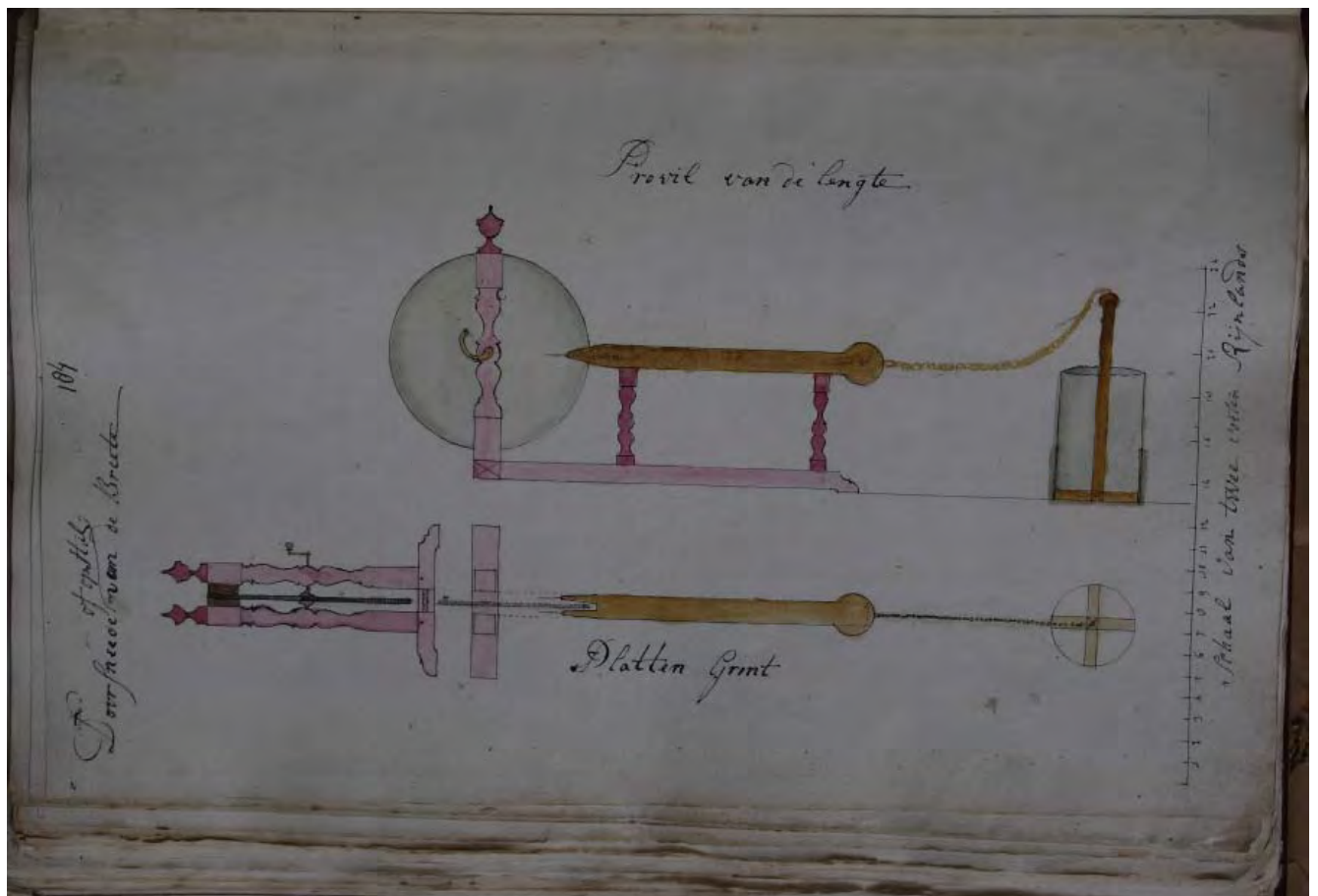
Ongedateerde tekening van een elektriseermachine door Hendrik Verhees. Tevens is onbekend waar, of naar welk voorbeeld de tekening werd gemaakt
