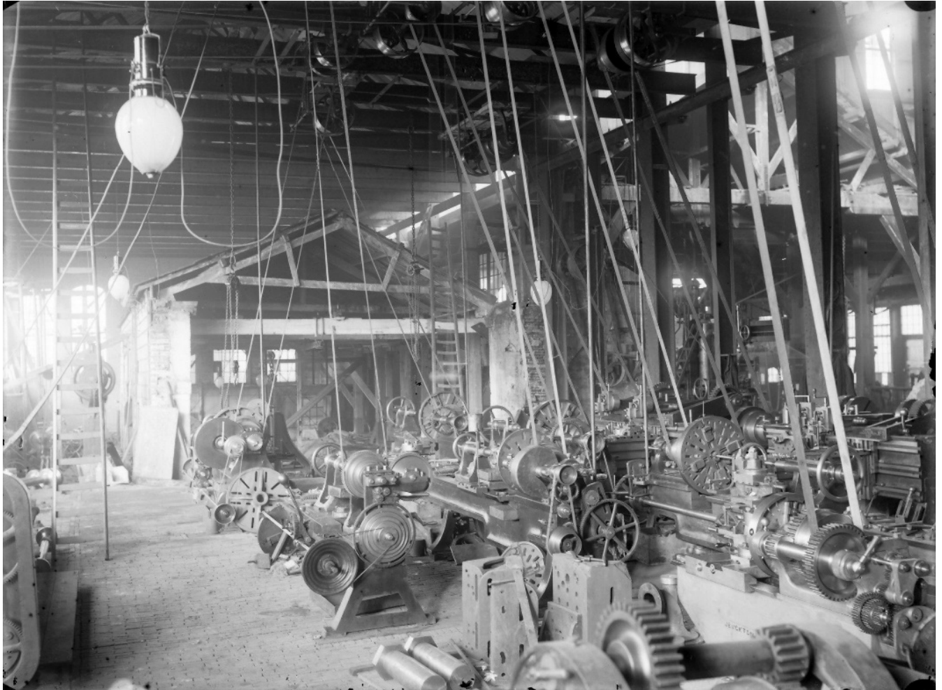
Fabrieksverlichting d.m.v. spitsbooglampen ca. 1881-1888 ( www.willemsmithistorie.nl )
