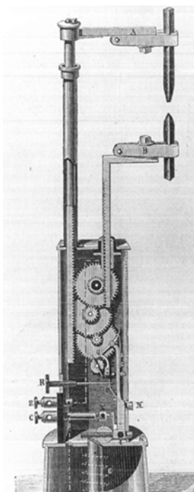
Principe werking spitsbooglamp
