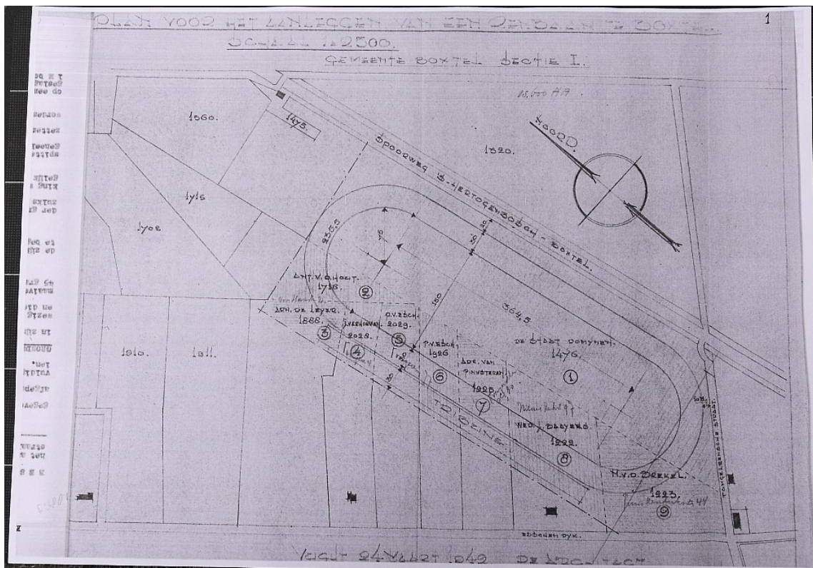
Tekening met als titel Plan voor het aanleggen van een Renbaan te Boxtel. Prominent is ook vermeld: Gemeente Boxtel. De Datum: 24 maart 1942. De tribune ligt tegenover de spoorlijn. De huidige straat Essche Heike wordt hier aangeduid met Tongerenschestraat. De renbaan uit de jaren veertig is meer richting Essche Heike gesitueerd dan de oorspronkelijk baan en is waarschijnlijk een stuk groter.
