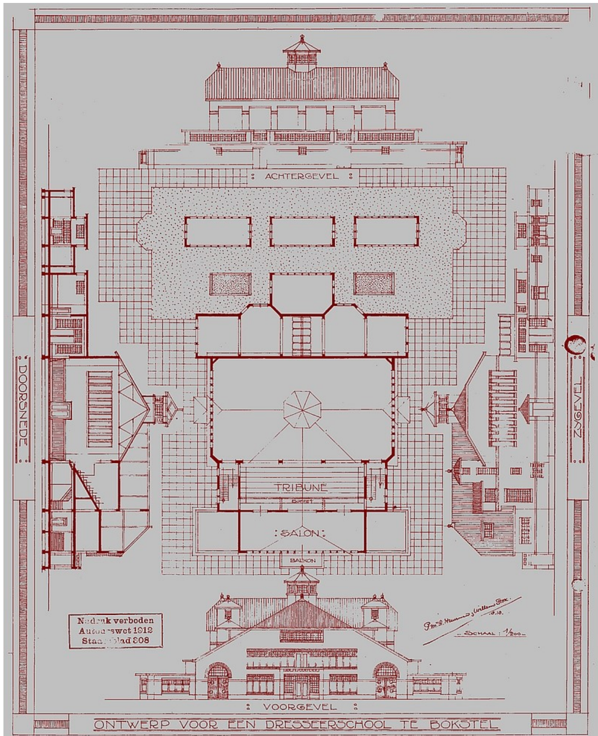
Ontwerp voor een hippisch centrum in Bokstel
