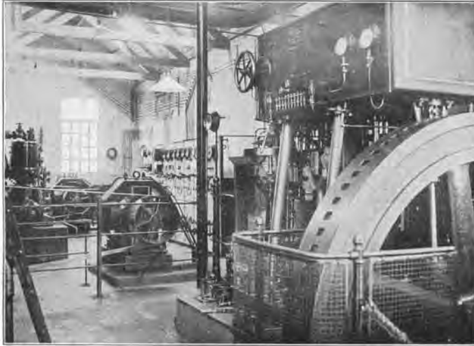
Een hoekje der machinekamer van de Electricische Centrale.
