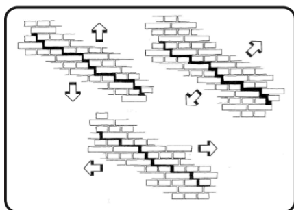
Scheurvorming in baksteen muren die aangeeft in welke richting krachten werken door scheurbreedteverschillen van lint- en stootvoeg!
